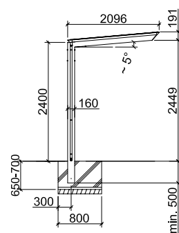
Seitenansicht Smart-Port
