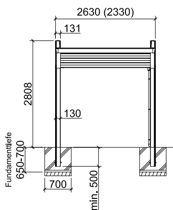
Vorderansicht Typ 60
