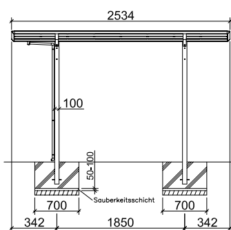
Vorderansicht Smart-Port
