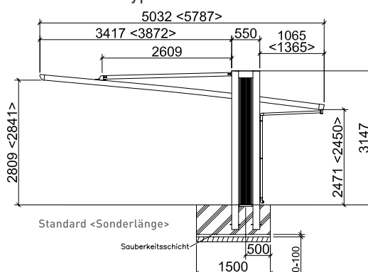
Seitenansicht Typ 150
