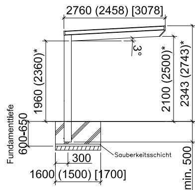
Vorderansicht
