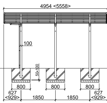
Standard <Sonderlänge>
