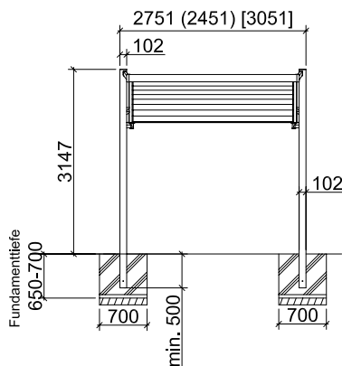
Vorderansicht Typ 150
