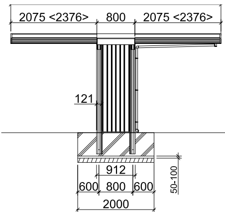
Seitenansicht
