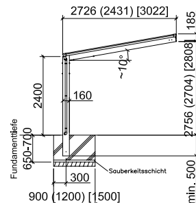
Seitenansicht Typ 110
