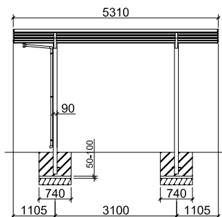
Vorderansicht Swingline
