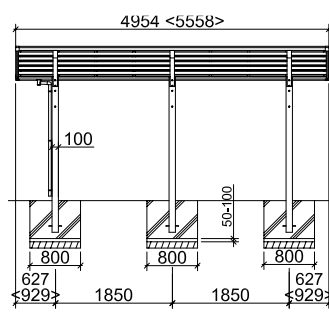
Vorderansicht Typ 110 (hat 3 Pfosten)
