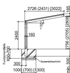
Seitenansicht Typen 60 – 80
