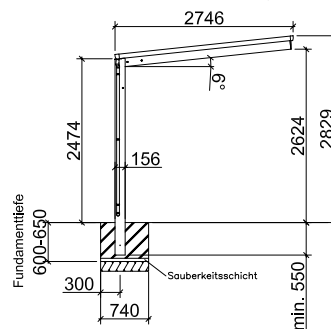
Seitenansicht Swingline
